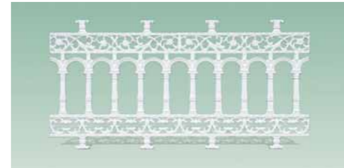
M 203 A)W1000×H570×T10, B)W1000×H548×T11 C)W1000×H500×T10, D)W1000×H400×T10, (다릿발이 별도로 없음)
