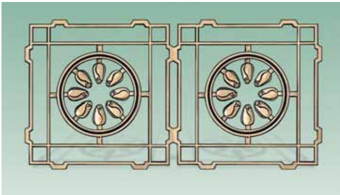
M 101 W200×H400×T9
