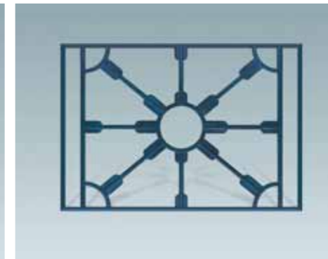
AF 863 W1160×H805×T17
