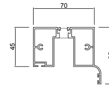
<상부프레임>
