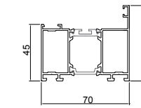
<문짝바>
