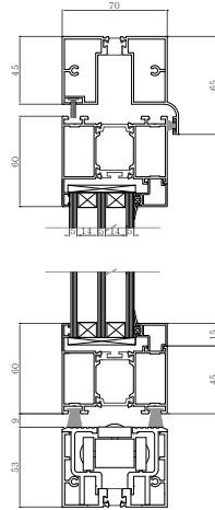
• 수직단면 상세도
