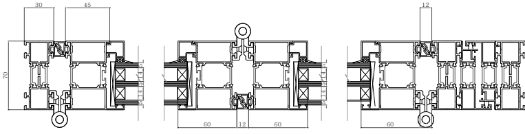
• 수평단면 상세도
