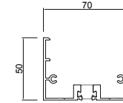
<하부프레임>
