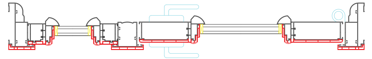
조립도 도면
