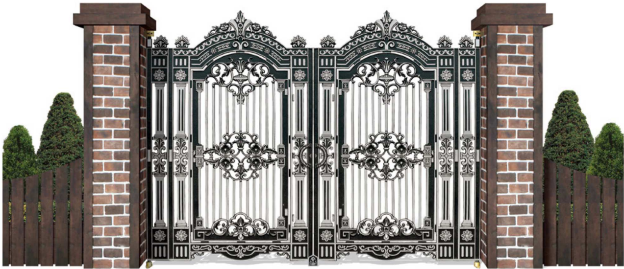
7034 대:W1200XH2125(한지시공높이 2000), 쪽문가능 중:W1200XH1780(한지시공높이 1650), 쪽문가능 소:W1200XH1500(한지시공높이 1350), 쪽문가능
