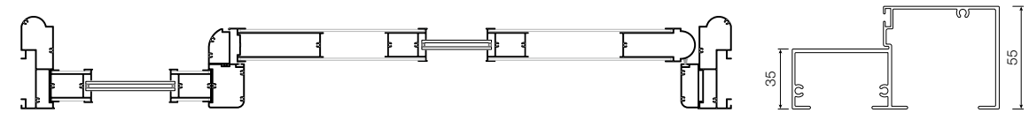
후레임 130mm | 문짝 47mm
