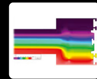
열관류율 해석
